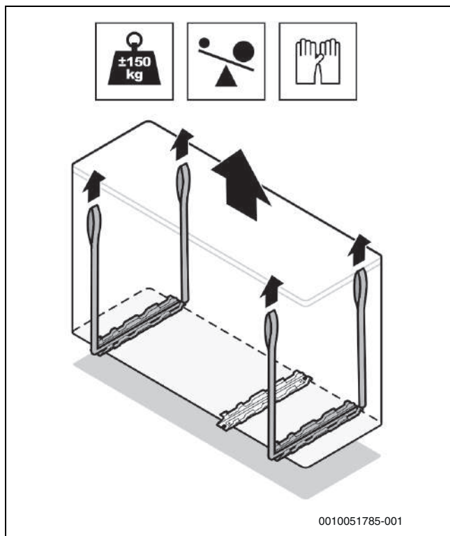
45. ábra Az egység elhelyezése
