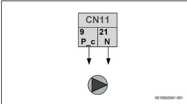
85. ábra 2. zóna keverőszivattyú, 2. típusú vezérlőjel
