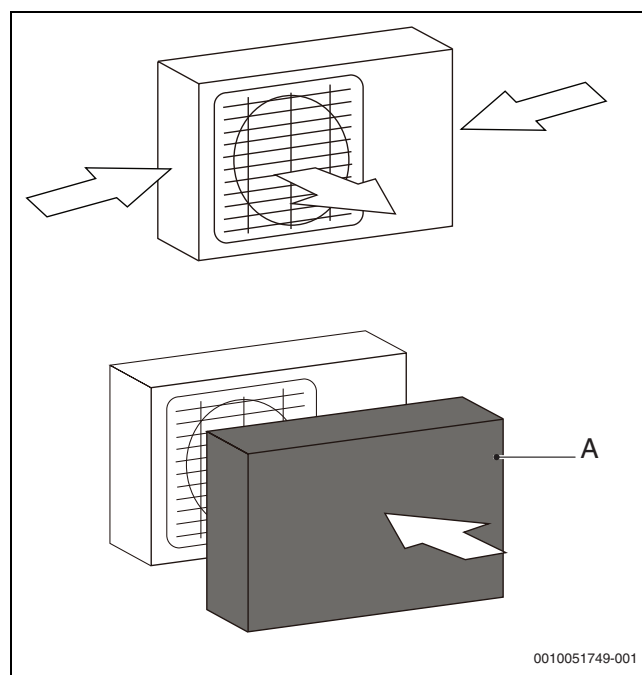
37. ábra Védje az egységet a különösen erős szélről.
