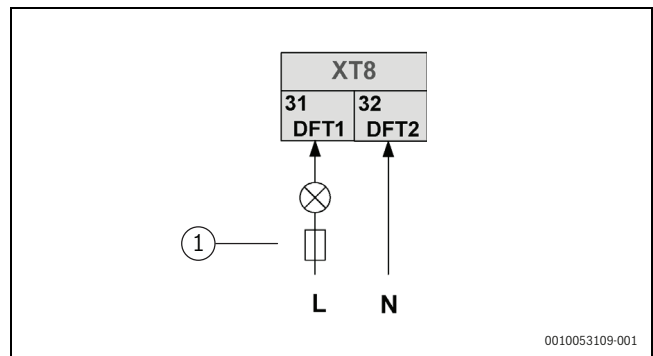
90. ábra Leolvasztási állapot vagy riasztási állapot
