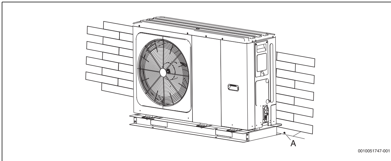
35. ábra A CS2000AWF 4 R-S ~ CS2000AWF 30 R-T egységek normál telepítése
