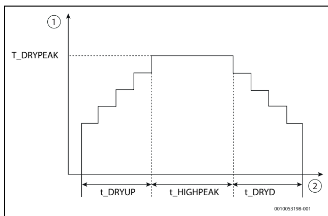
143. ábra Esztich-száritási ciklus diagram
