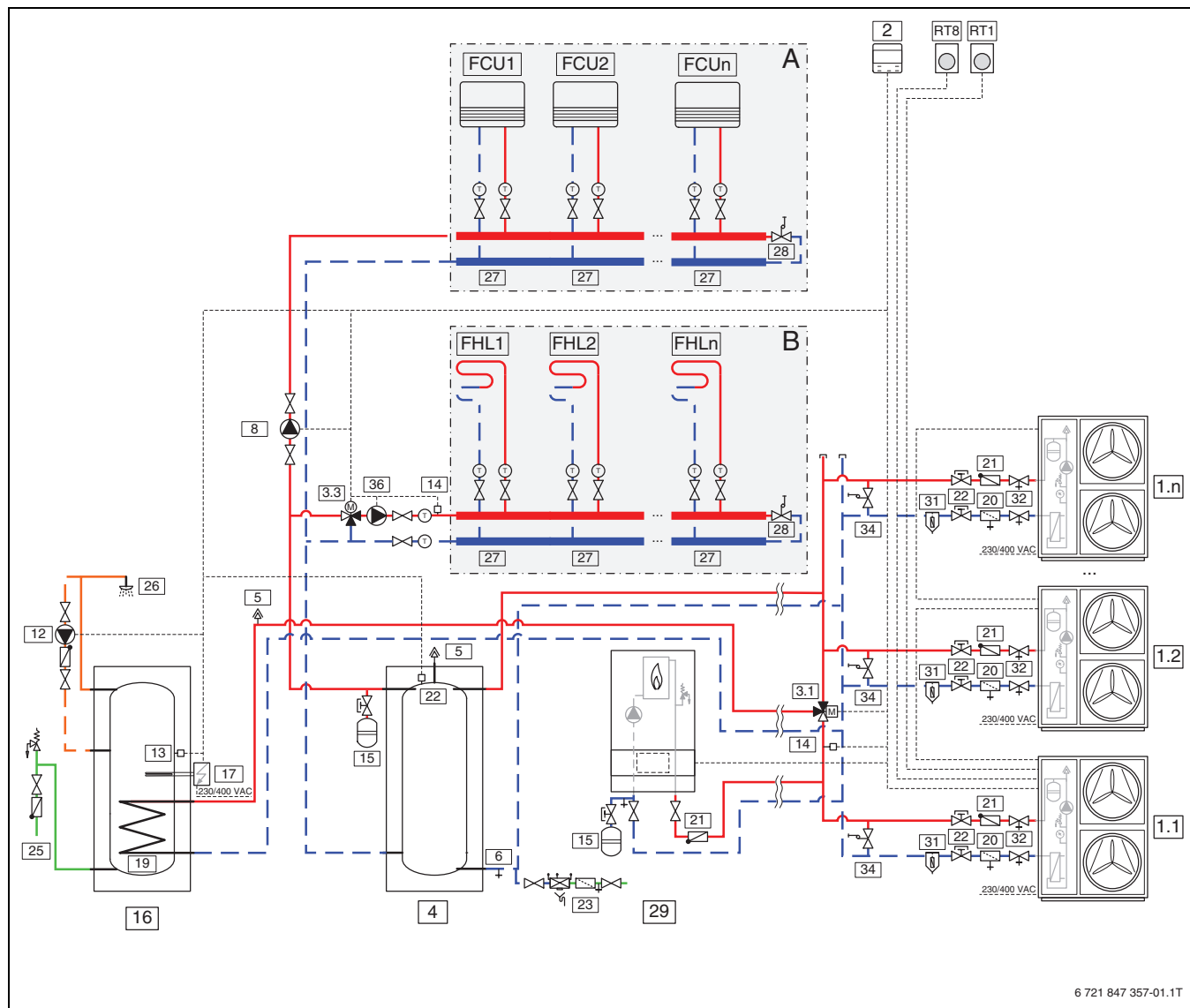
27. ábra Kültéri egység egy vagy több fűtőkörrel, külső kiegészítő fűtőberendezéssel, melegvíz-tárolóval és kaszkádrendszerrel (CS2000AWF 18 -30 R-T)
