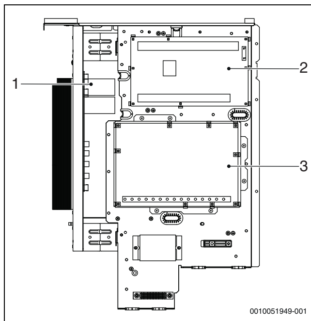
63. ábra CS2000AWF 18 R-T és CS2000AWF 16 R-S/CS2000AWF 30 R-T közötti méretek
