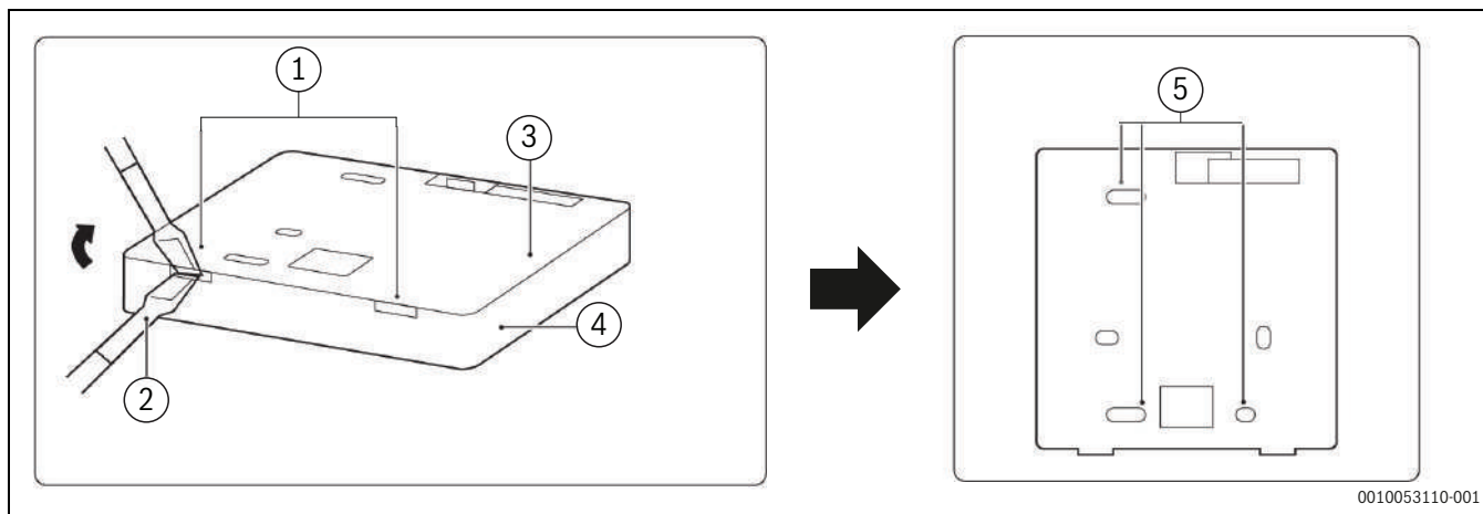
97. ábra Falra szerelés
