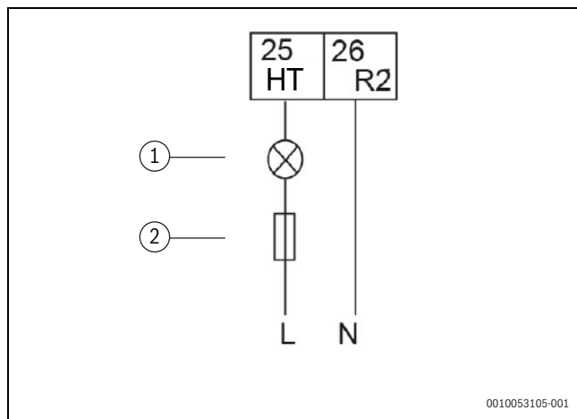
74. ábra 1. TÍPUSÚ vezérlőjel
