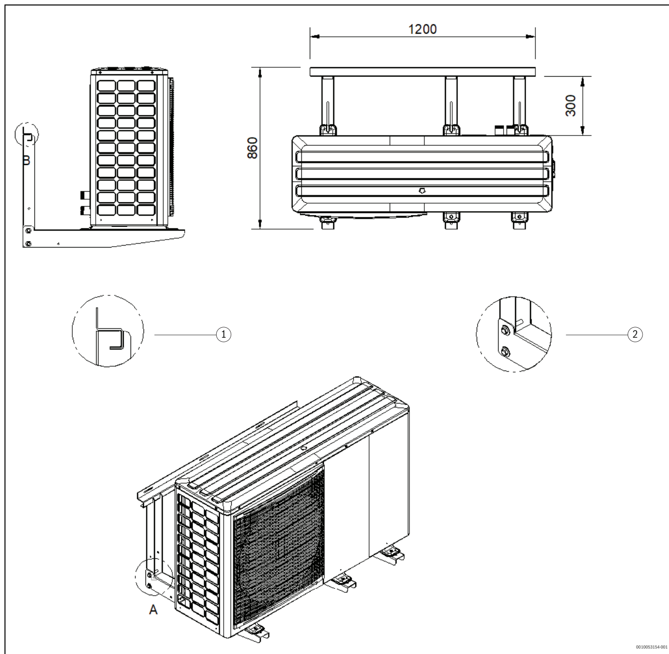
44. ábra Falra szerelés
