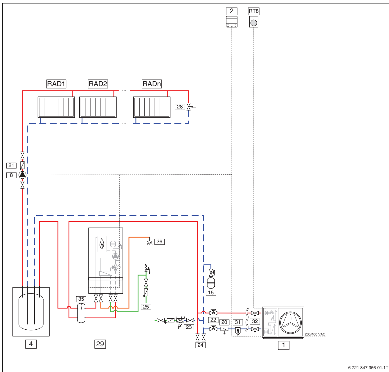
26. ábra Kültéri egység egy vagy több fűtőkörrel és külső kiegészítő fűtőberendezéssel (CS2000AWF 4-6 R-S, CS2000AWF 8-10 R-S, CS2000AWF 12-16 R-S/T)
