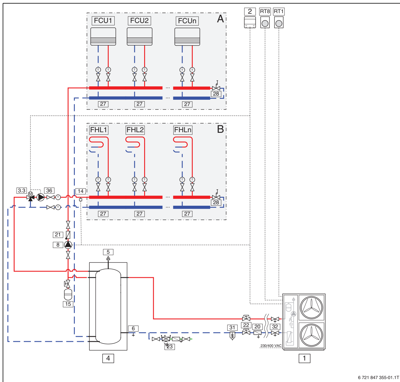
25. ábra Kültéri egység egy vagy több fűtőkörrel, padlófűtéssel és radiátorokkal (CS2000AWF 18-30 R-T)
