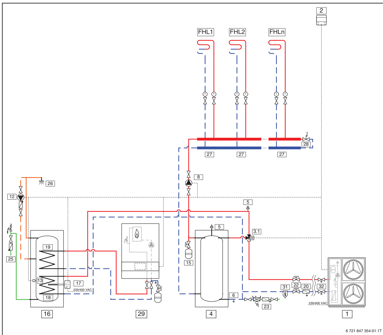
24. ábra Külső egység egy vagy több fűtőkörrel, külső kiegészítő fűtőberendezéssel és melegvíz-tárolóval (CS2000AWF 18-30 R-T)
