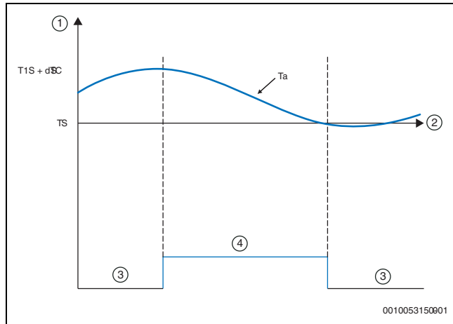
123. ábra Hűtési üzem – Levegő hőmérséklete ( T_a )
