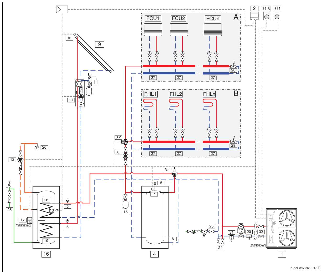
21. ábra Kültéri egység egy vagy több fűtőkörrel, tartalék elektromos fűtőberendezéssel, melegvíz-tárolóval és napkollektorral (CS2000AWF 18-30 R-T)
