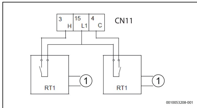
103. ábra Zóna termosztát – C módszer
