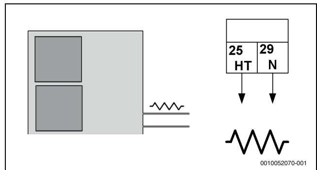
91. ábra Fagymentesítő fűtőberendezés csövekhez
