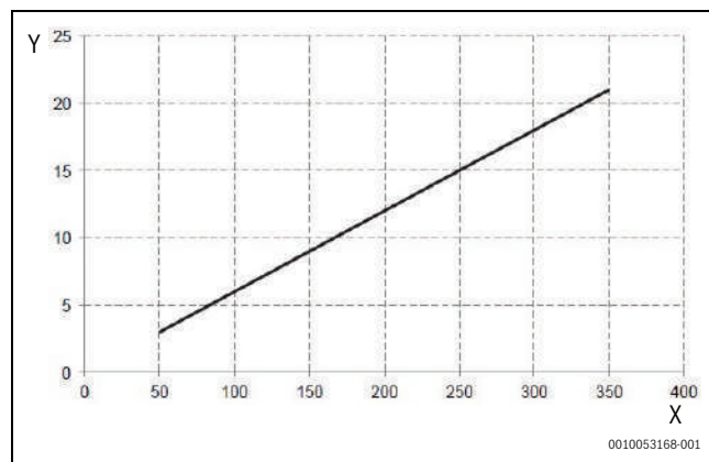
56. ábra A tágulási tartály teljes térfogata (CS2000AWF 4 R-S és CS2000AWF 16 R-S/CS2000AWF 16 R-T közötti méretek)
