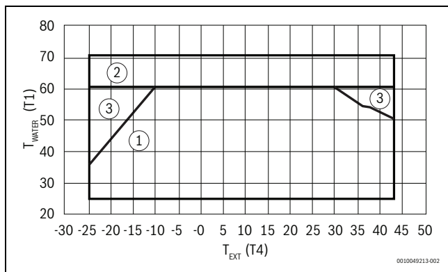
10. ábra CS2000AWF 18-30 R-T
