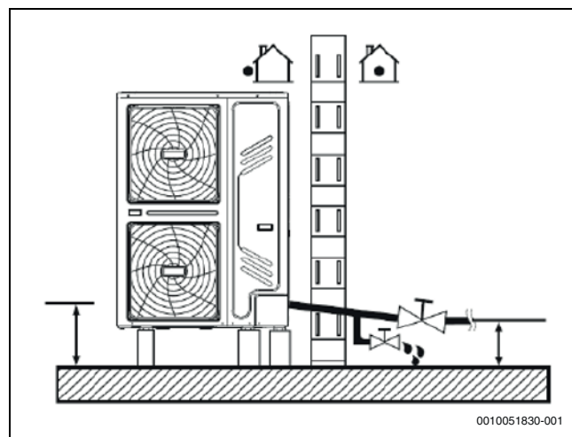
54. ábra A vízkör fagyvédelme
