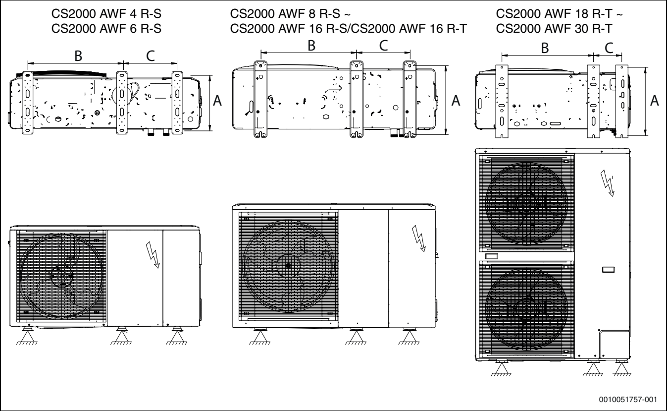
42. ábra Méretek földre rögzítéshez
