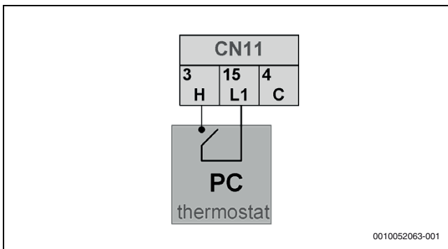
87. ábra Helyiség termosztát HMI konfiguráció
