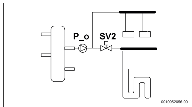
81. ábra Dupla zónás rendszer
