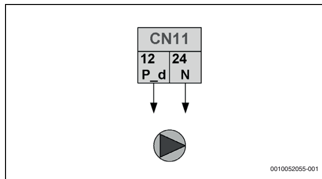
80. ábra Melegvíz-szivattyú, 2. típusú vezérlőjel
