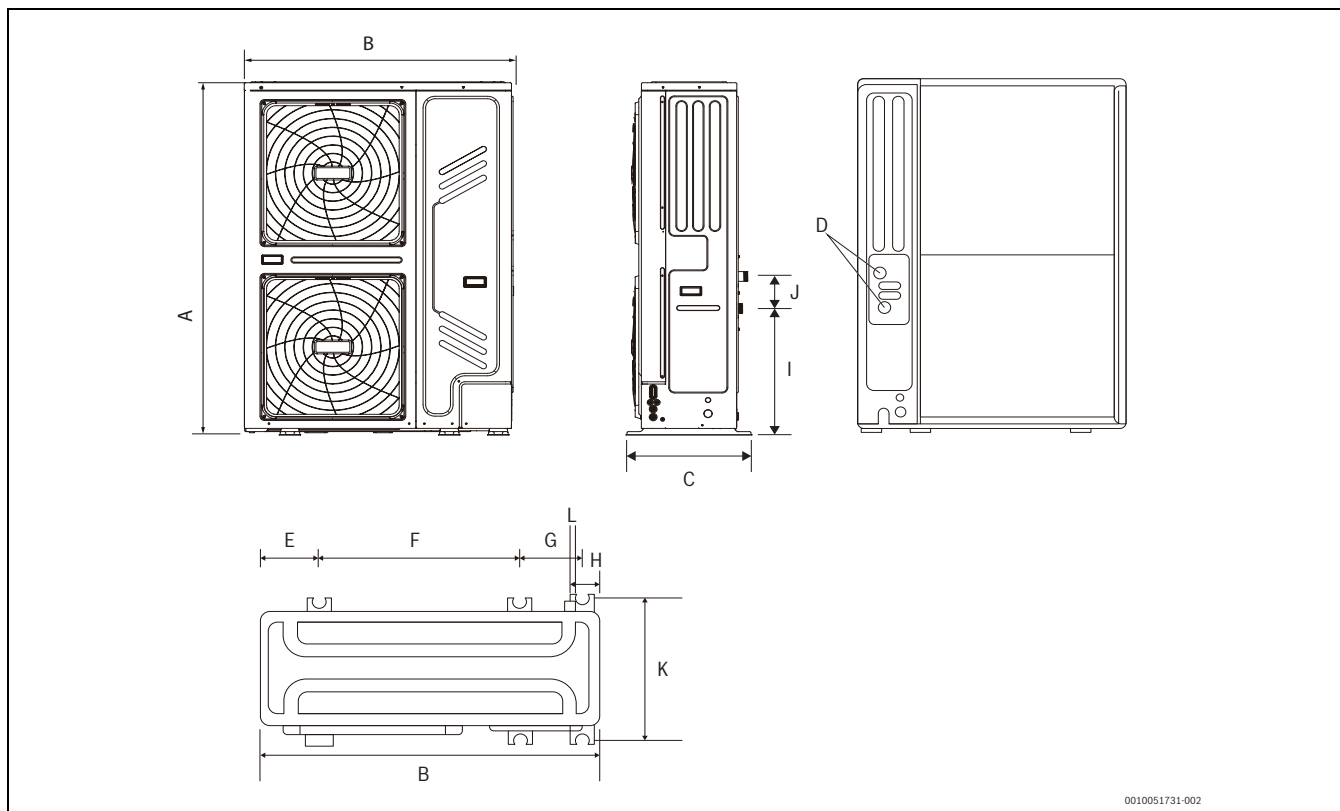
34. ábra CS2000AWF 18 R-T és CS2000AWF 30 R-T közötti méretek
