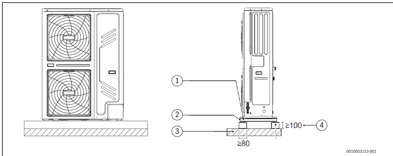
43. ábra Rögzítse az egységet alapozócsavarokkal
