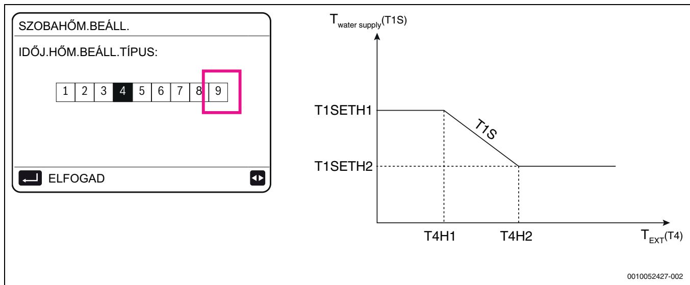
147. ábra Testre szabható görbe – külső levegő hőmérséklete ( T_{4H1} , T_{4H2} ) és vízhozzávezetés ( T_{1SETH1} , T_{1SETH2} )
