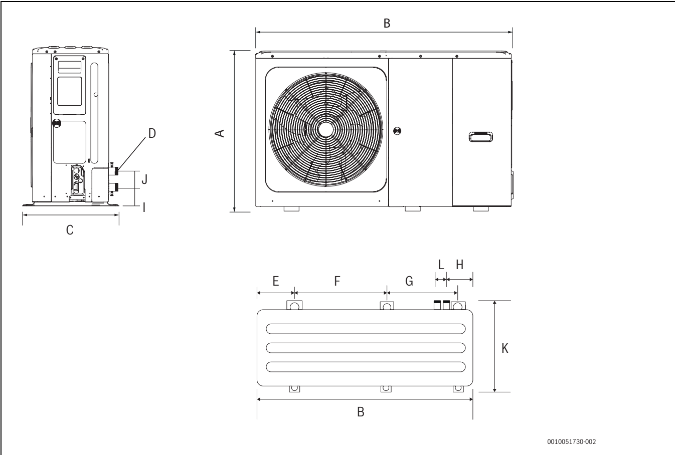
33. ábra CS2000AWF 8 R-S és CS2000AWF 16 R-S/CS2000AWF 16 R-T közötti méretek
