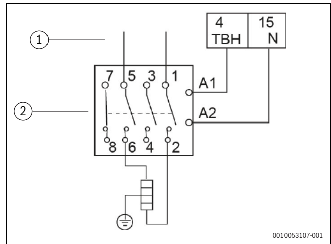
75. ábra 2. TÍPUSÚ vezérlőjel
