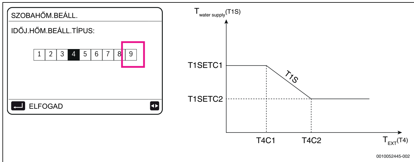
150. ábra Testre szabható görbe – külső levegő hőmérséklete ( T_{4C1} , T_{4C2} ) és vízhozzávetés ( T_{1SETC1} , T_{1SETC2} )
