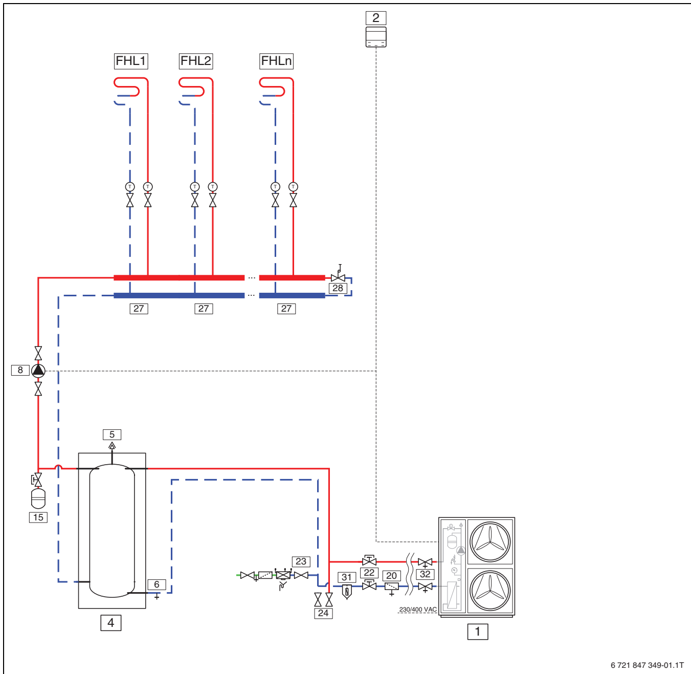
19. ábra Kültéri egység egy vagy több fűtőkörrel (CS2000AWF 18-30 R-T)
