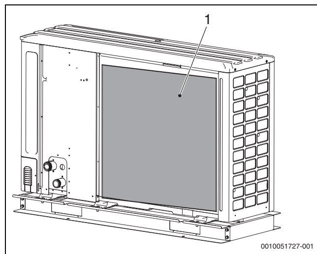
30. ábra A csomagolás eltávolítása
