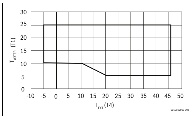
12. ábra CS2000AWF 18-30 R-T
