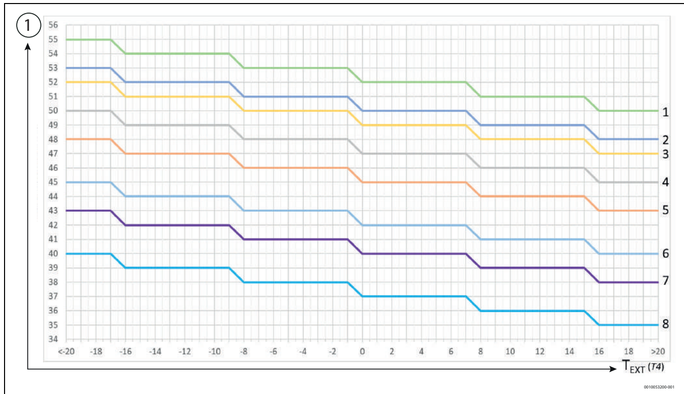
146. ábra Fűtési üzem végponti elosztással rendelkező rendszerekben
