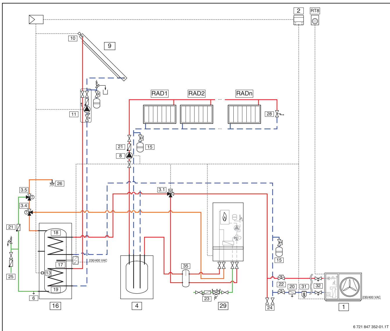
22. ábra Kültéri egység egy vagy több fűtőkörrel, külső kiegészítő fűtőberendezéssel, melegvíz-tárolóval és napkollektorra (CS2000AWF 4-6 R-S, CS2000AWF 8-10 R-S, CS2000AWF 12-16 R-S/T)
