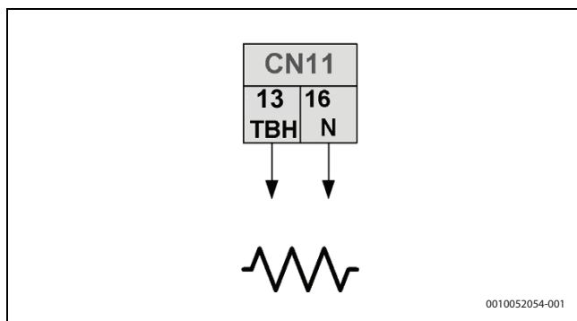
79. ábra Elektromos fűtőbetét kábel HMI konfiguráció, 2. típusú vezérlőjel
