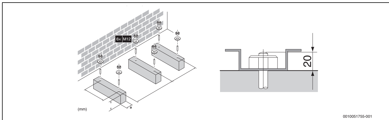
41. ábra Földre szerelés
