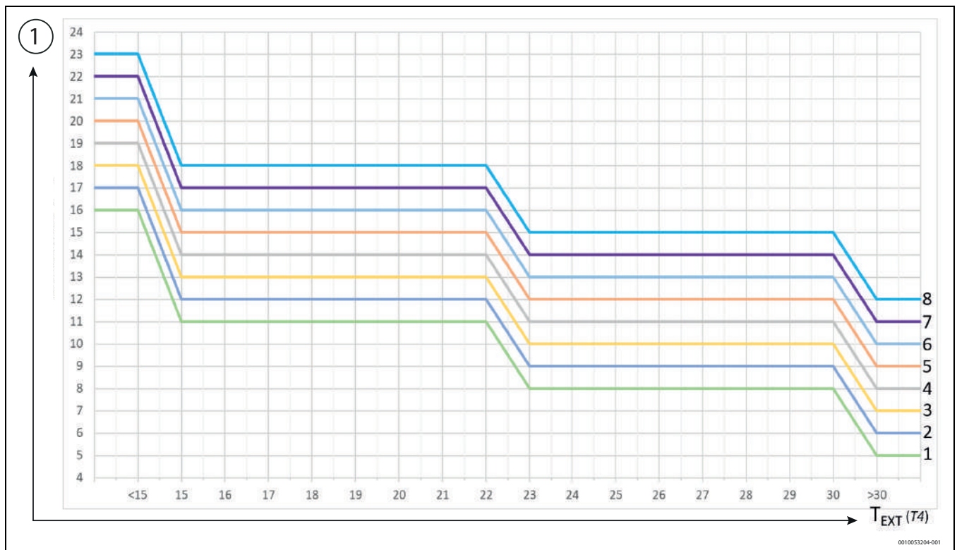
149. ábra Hűtési üzem végponti elosztással rendelkező rendszerekben
