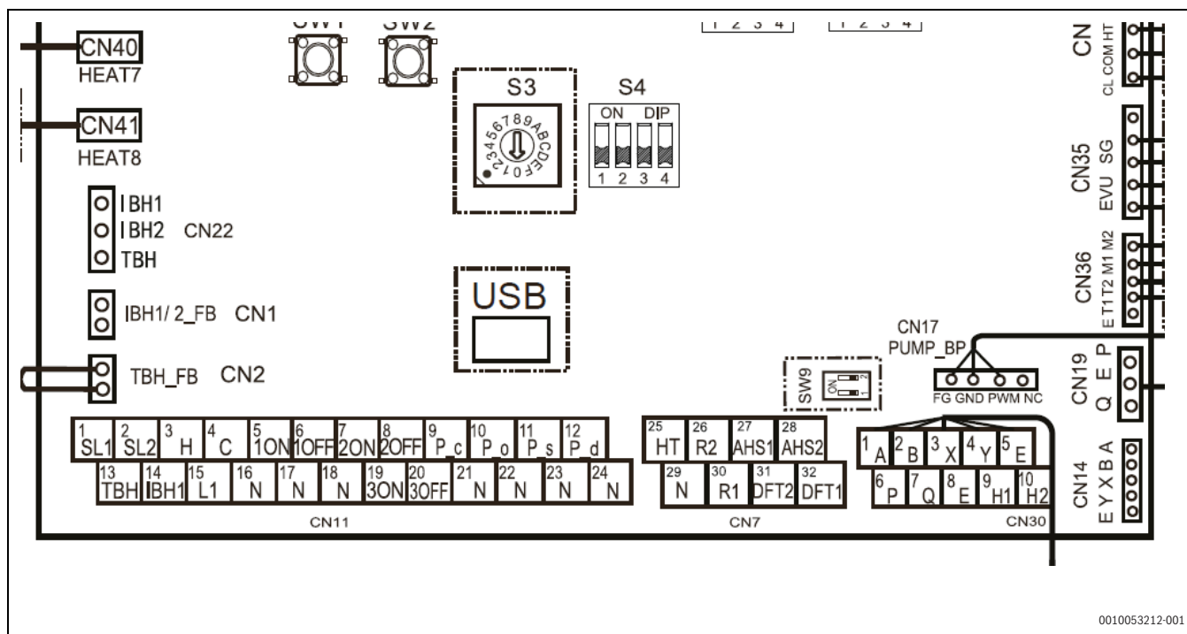
73. ábra Sorkapocslec csatlakoztatása
