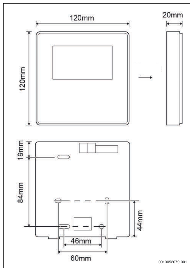
95. ábra A felhasználói felület beszerelése
