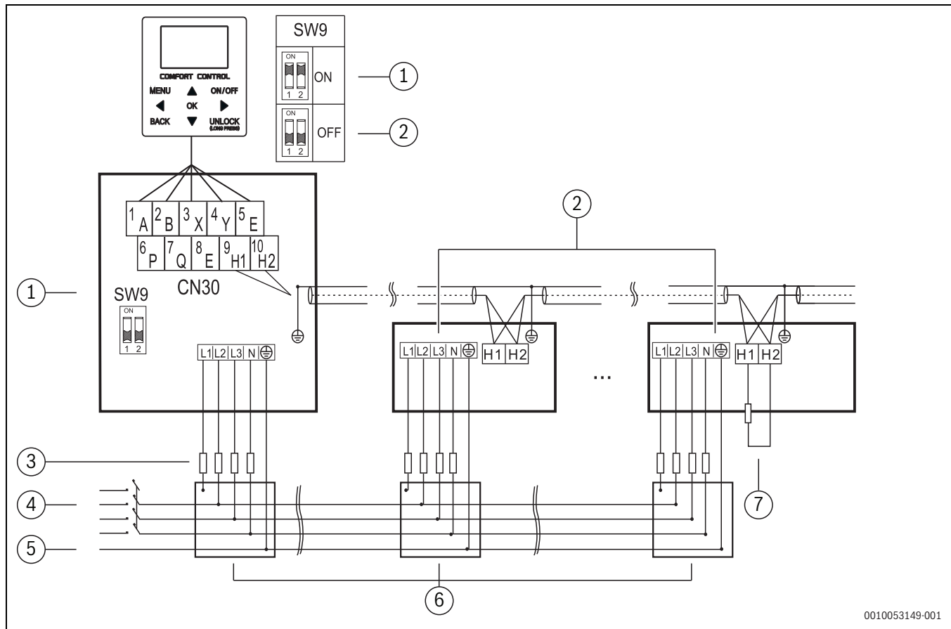
68. ábra A kaskádrendszer elektromos vezérlőrendszerének kapcsolási rajza (3 N ~)
