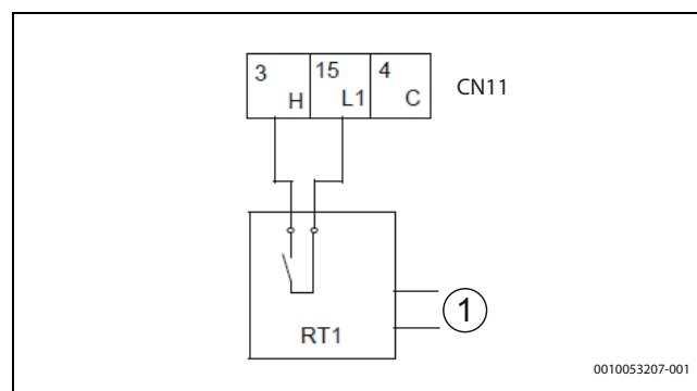
102. ábra Zóna termosztát – B módszer
