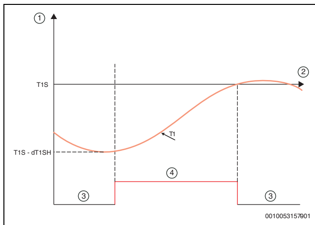
125. ábra Fűtési üzem – Előremenővíz- hőmérséklete (T1)
