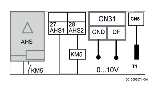
92. ábra Kiegészítő kazán
