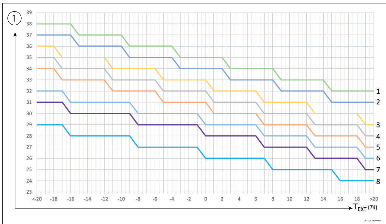
145. ábra Fűtési üzem padlófűtéssel rendelkező rendszerekben
