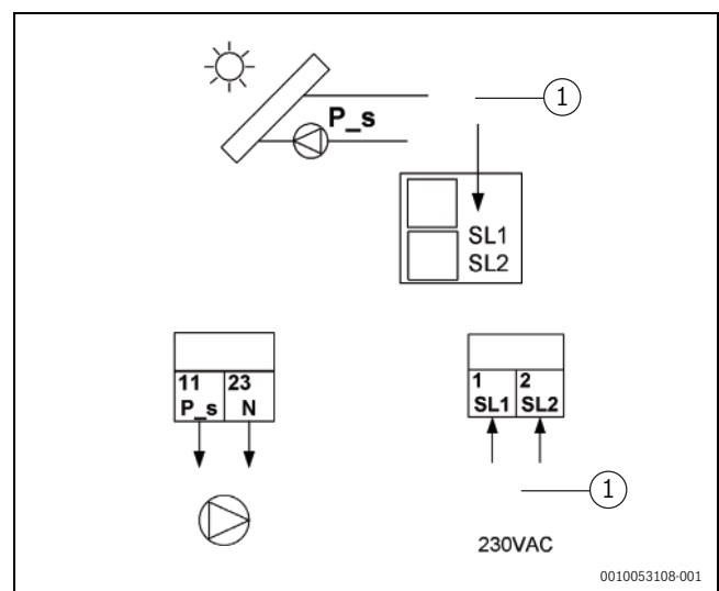
76. ábra Szolár / Szolárzivattyú HMI konfiguráció
