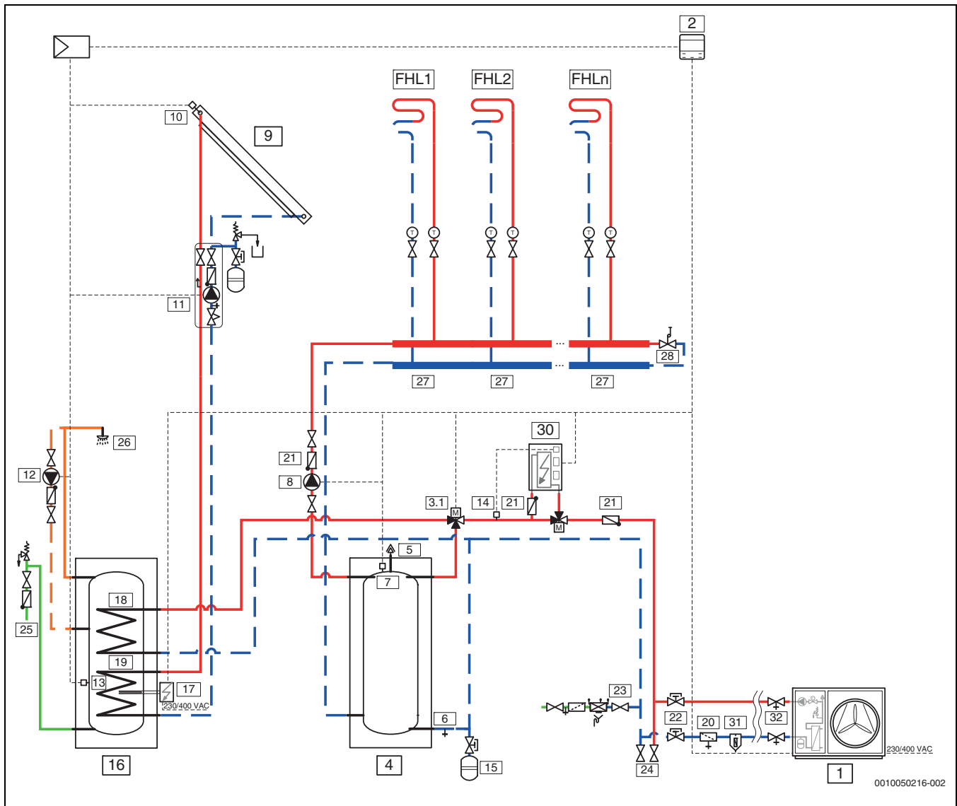
15. ábra Kültéri egység egy vagy több fűtőkörrel, tartalék elektromos fűtőberendezéssel, melegvíz-tárolóval és napkollektorral (CS2000AWF 4-6 R-S, CS2000AWF 8-10 R-S, CS2000AWF 12-16 R-S/T)
