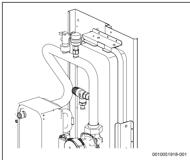
60. ábra Töltés / utántöltés vízzel
