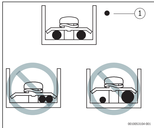
70. ábra Laza kábelezés esetén fennáll a túlmelegedés veszélye
