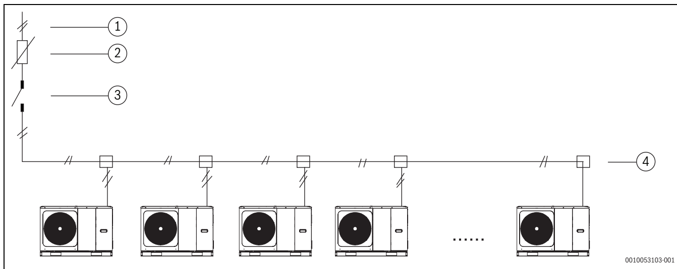
71. ábra Elektromos kör
