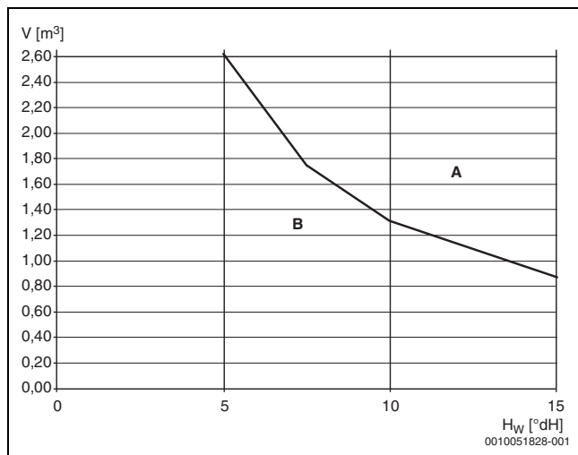
53. ábra A hőszivattyú < 50 kW teljesítményére vonatkozó előírt határértékek
