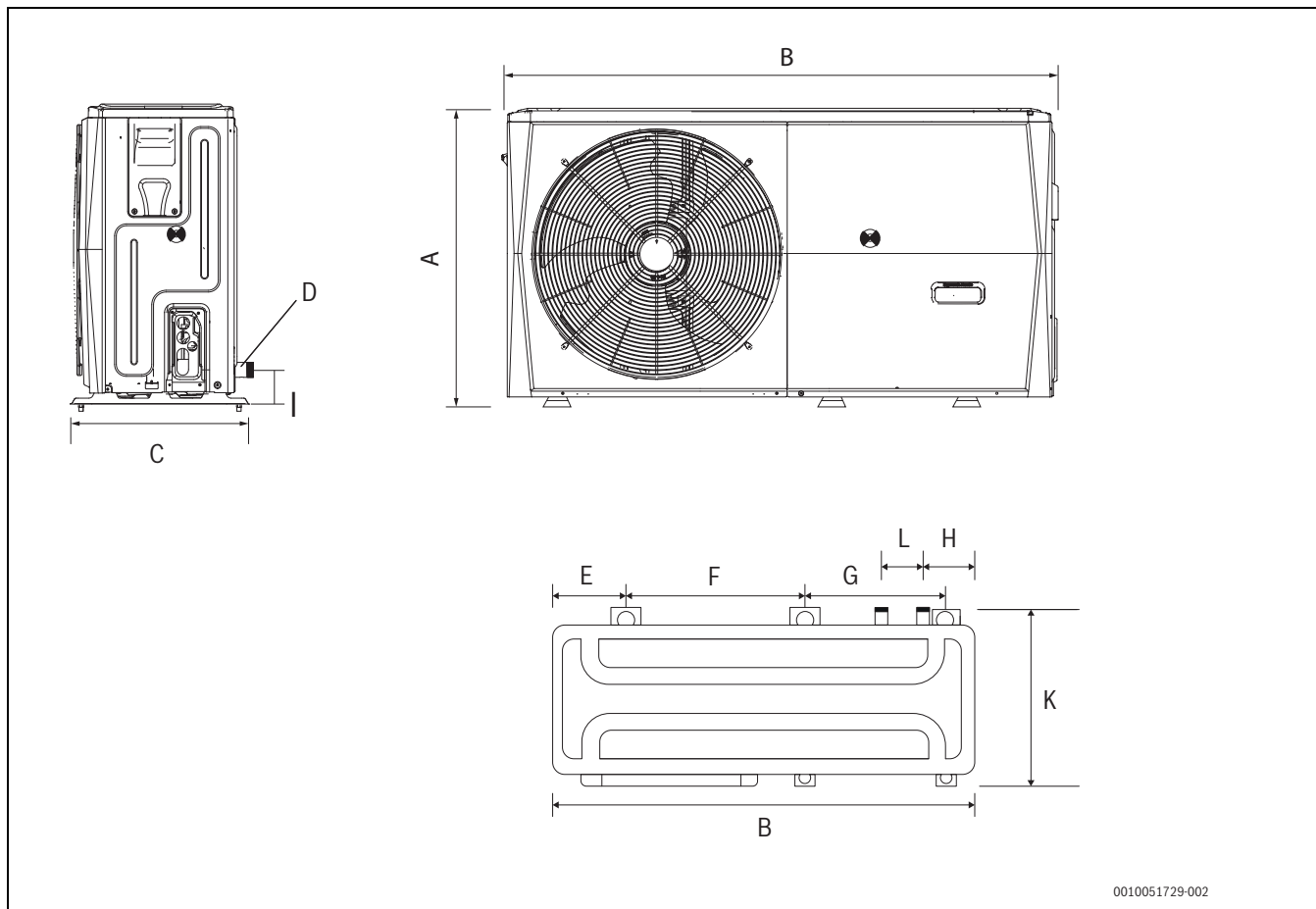
32. ábra CS2000AWF 4 R-S és CS2000AWF 6 R-S közötti méretek
