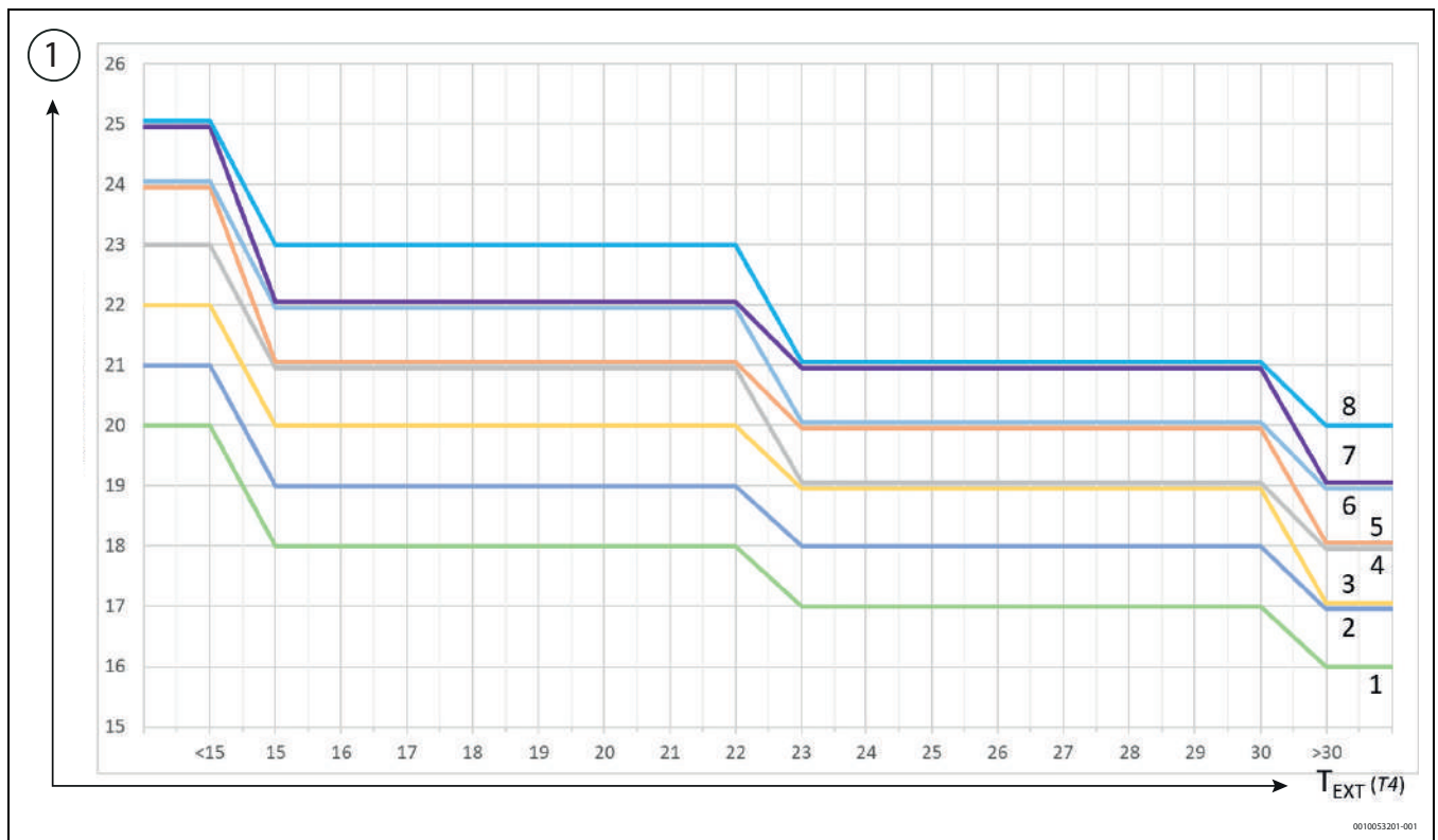
148. ábra Hűtési üzem padlófűtés-elosztással rendelkező rendszerekben
