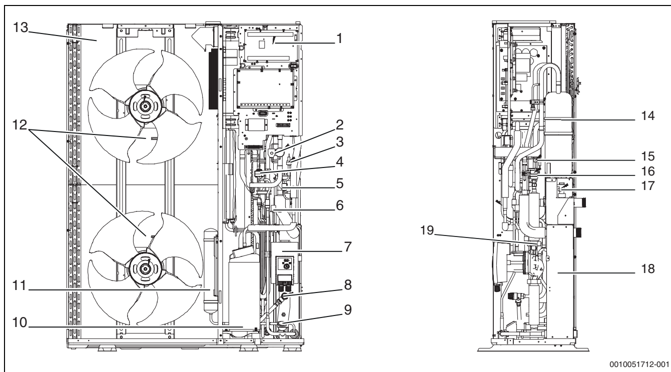
5. ábra CS2000AWF 18 R-T és CS2000AWF 30 R-T közötti méretek
