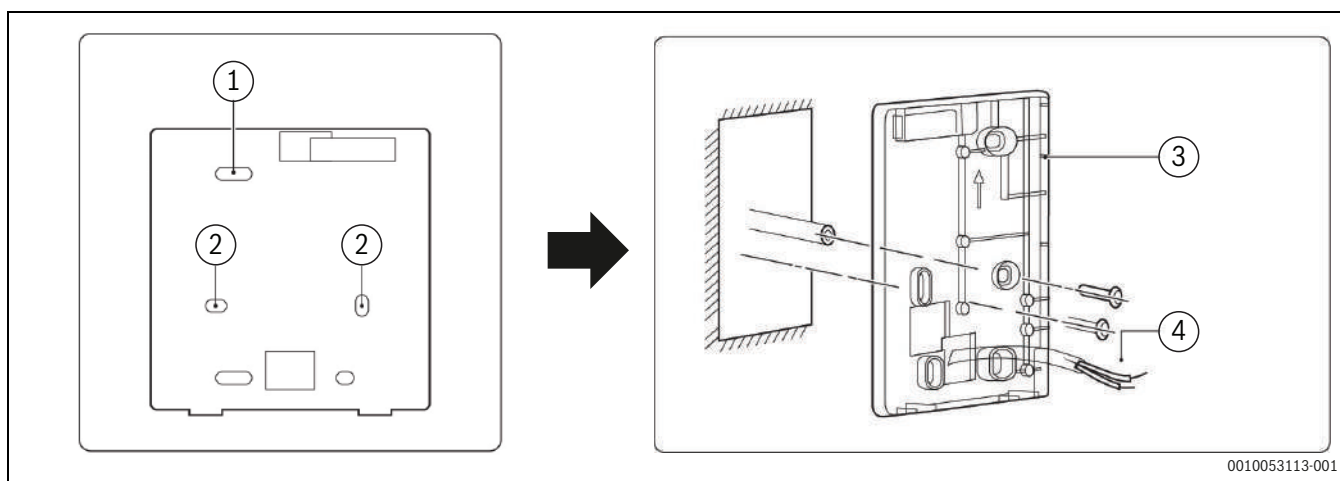
98. ábra Beszerelés a 86 kapcsolsszekrénybe
